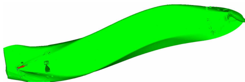
Fig.14.2 LNG carrier(B),H2(39),2.087Hz.
