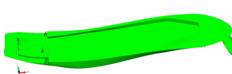
Fig.13.2 LNG carrier(F),H2(27),1.637Hz.
