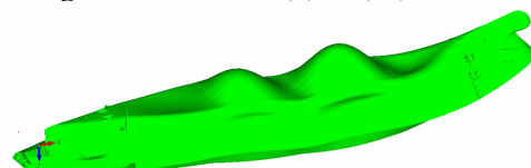
Fig.12.4 LNG carrier(B),V4(59),2.574Hz.
