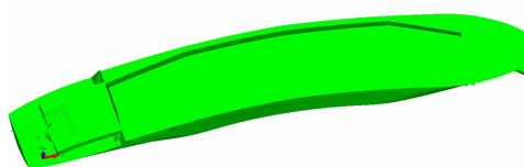
Fig.13.1 LNG carrier(F),H1(14),1.015Hz.
