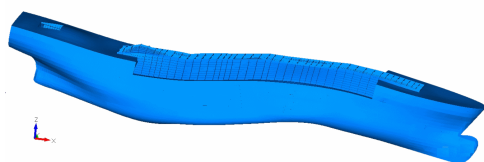
Fig.3.2 LPG carrier(F),V2(9),3.135Hz.
