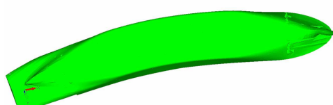
Fig.14.1 LNG carrier(B),H1(19),1.281Hz.
